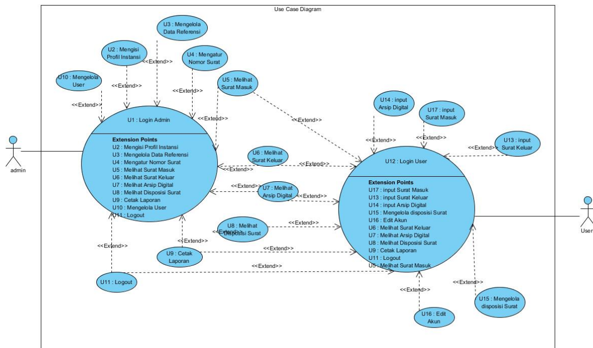
Gambar 3 Usecase Diagram Aplikasi Digital Archiving
