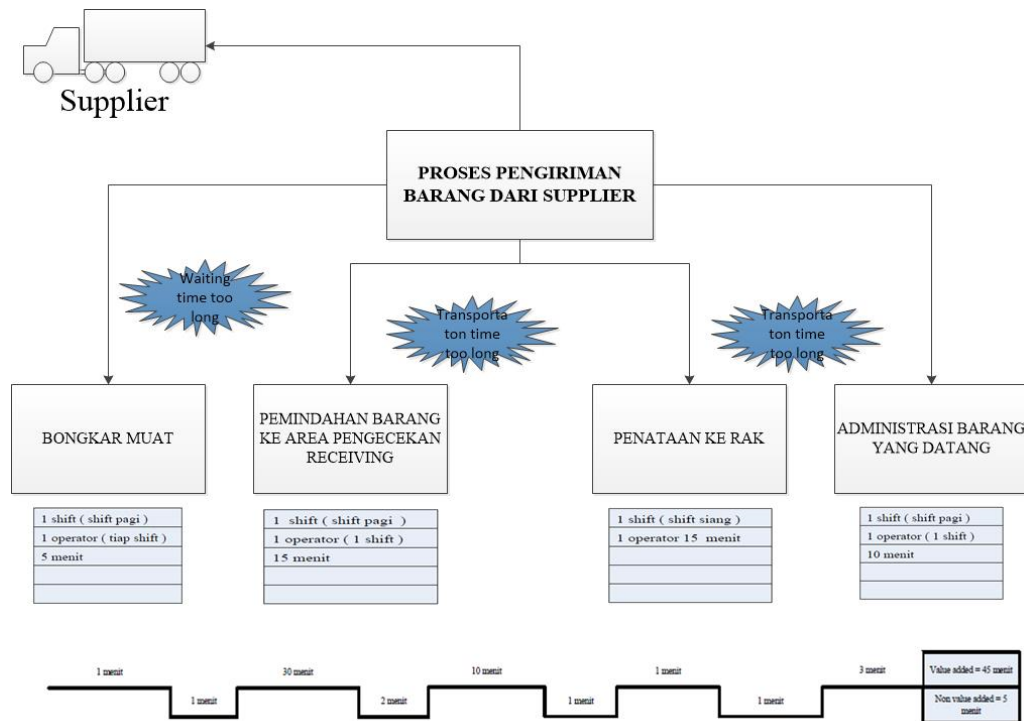
Gambar 5. Value Stream Mapping Pengiriman Barang dari Supplier
