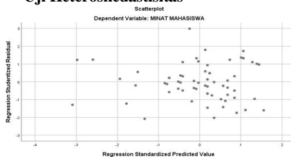
Gambar 1 Hasil Uji Heteroskedastisitas Scatterpot
